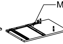
Middle plate :527x358x15=1
